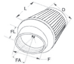
F - Diámetro inferior D - Diámetro del filtro L - Largo del filtro
